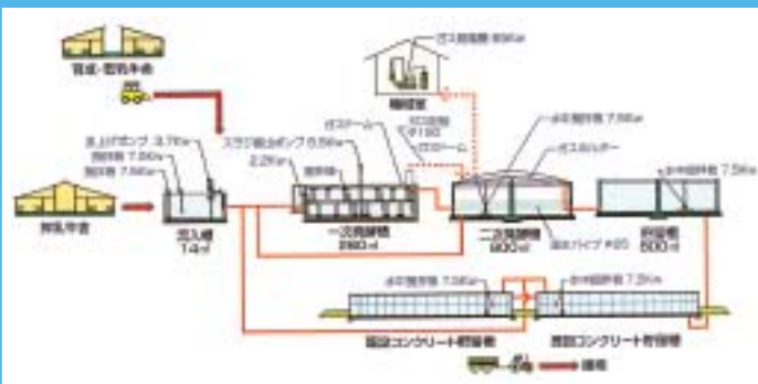
町村牧場バイオガスプラントの システムフロー (株)コーンズ・エーजीのパフレットより引用)
