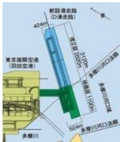
D滑走路完成イメージ図及びD滑走路平面図 (東京空港整備事務所資料)
