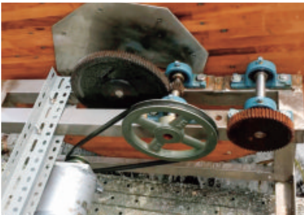
水車発電 (月寒川にぎわい川祭り)
