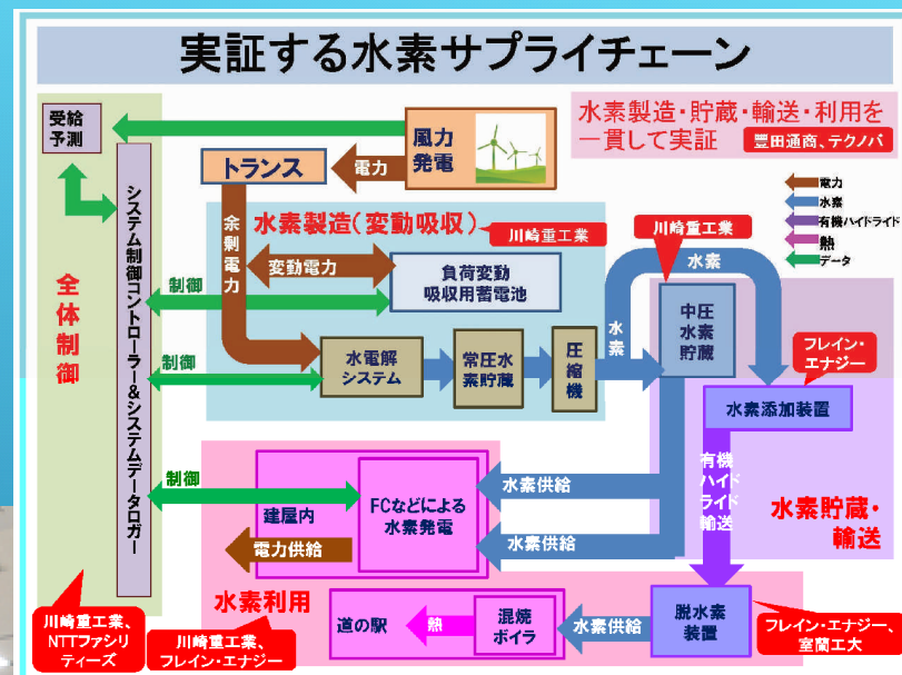
図-2 北海道苫前町で実証する水素サプライチェーン
