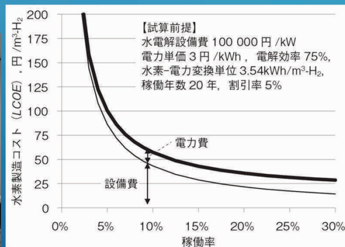
図. 設備費の影響と稼働率の関係(九州大学 土肥ほか 日本機械学会誌2016年4月より)
