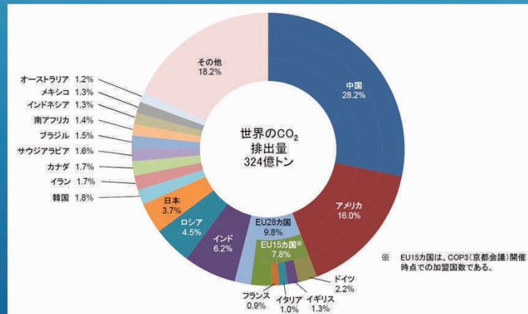
図. 世界のエネルギー起源CO 2 排出量2014
