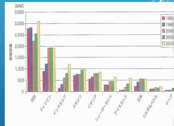
図. 主要地熱資源国の設備容量の推移
